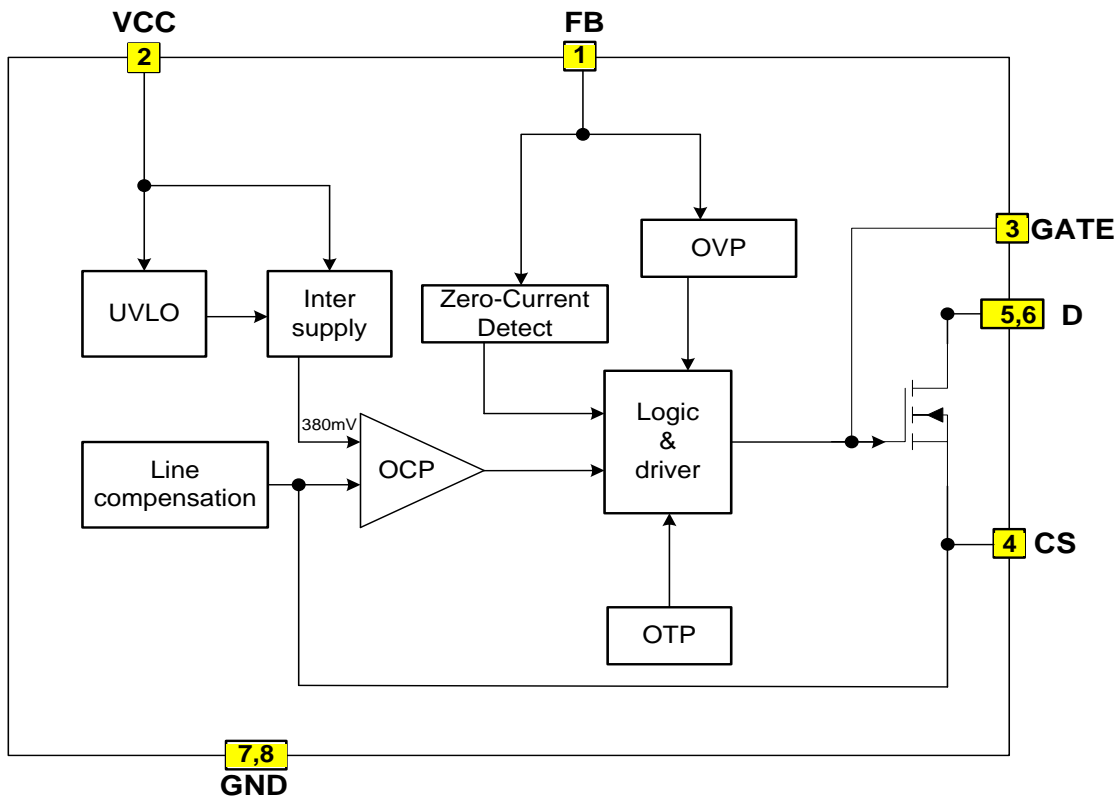
电路功能框图 (SP9135D)
