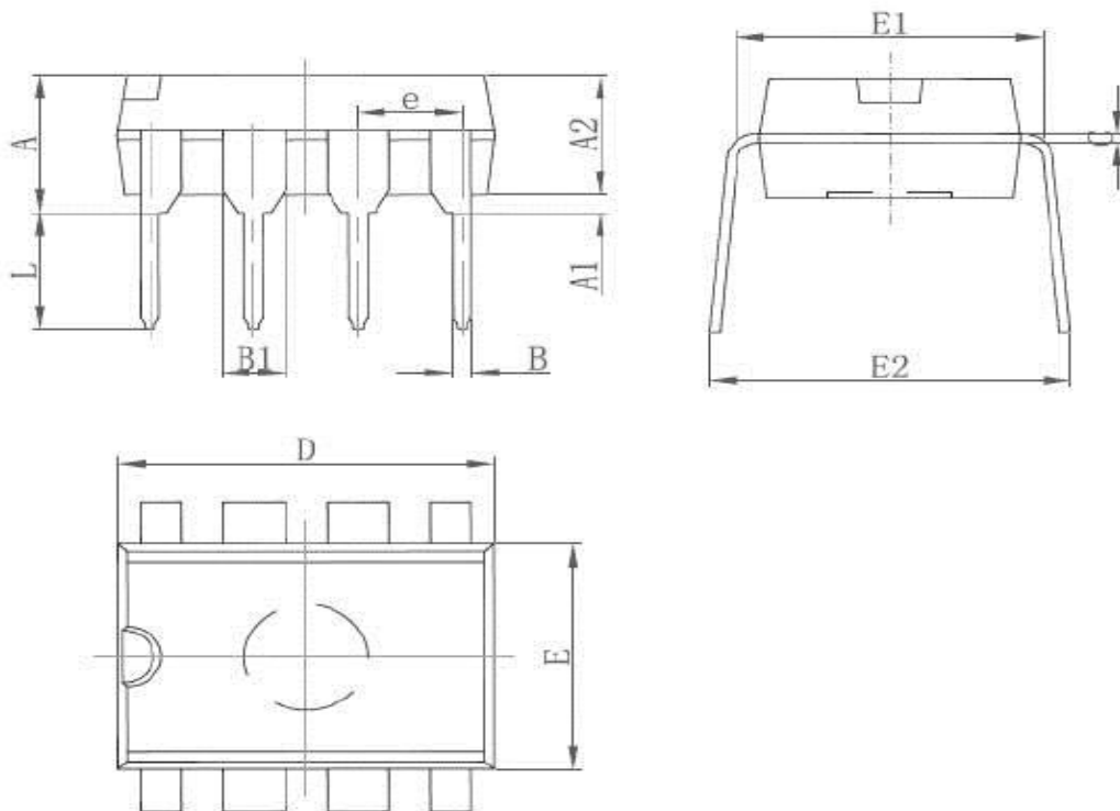
DIP8 封装外观图
